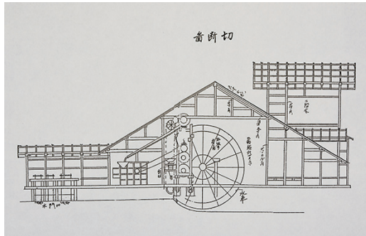
タマグルマ「断面図」
